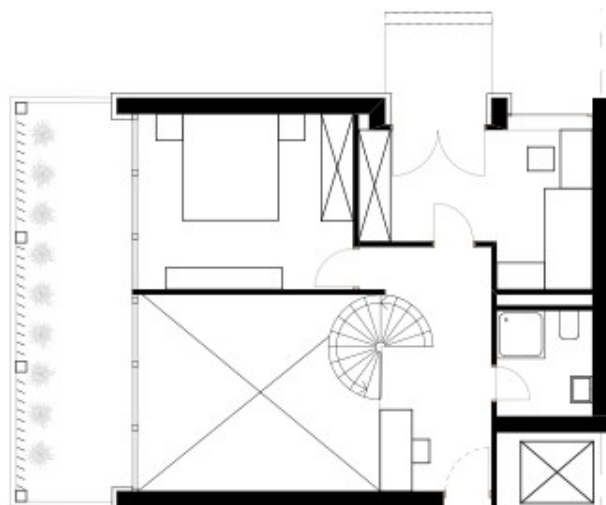
etaža 2
