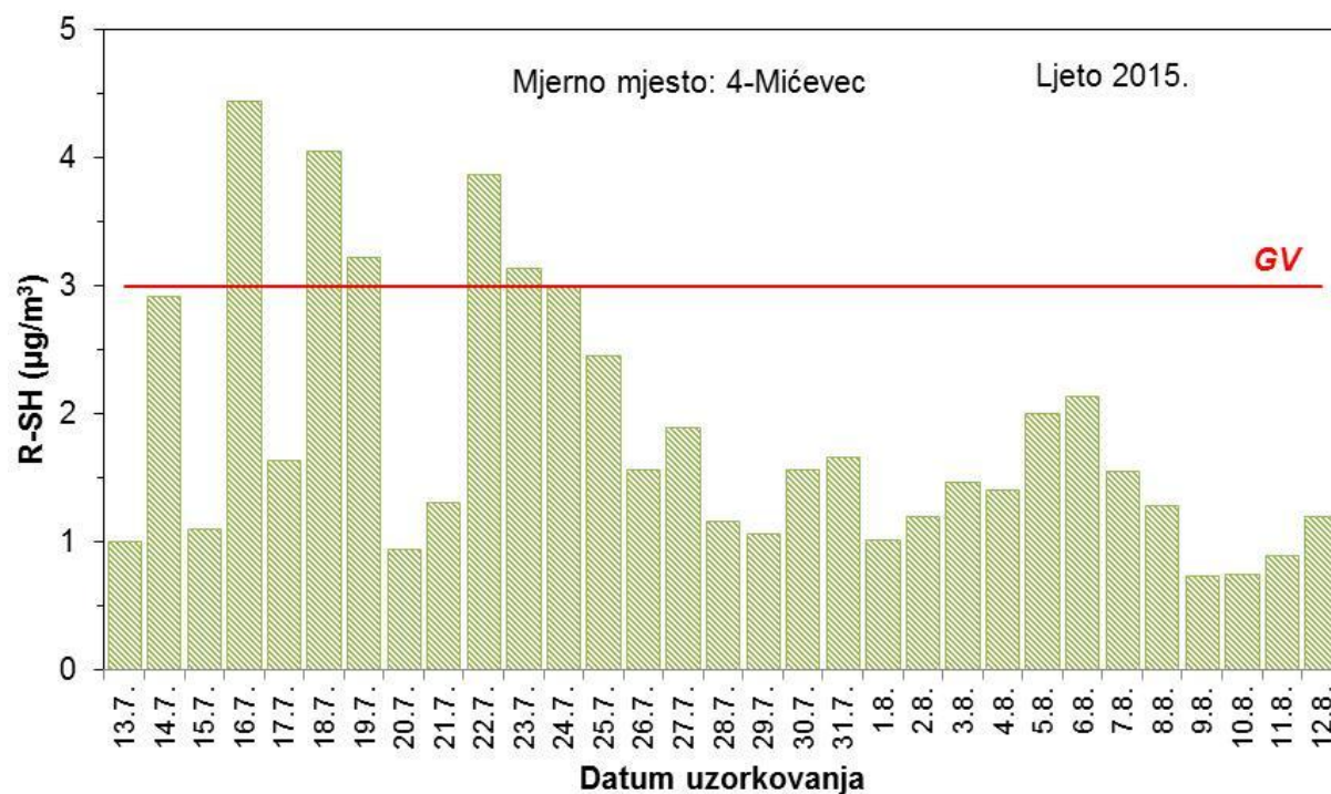
Slika 40 – Kretanje srednjih dnevnih koncentracija merkaptana na mjernoj postaji 4 – Mičevec tijekom ljetnog razdoblja mjerenja
