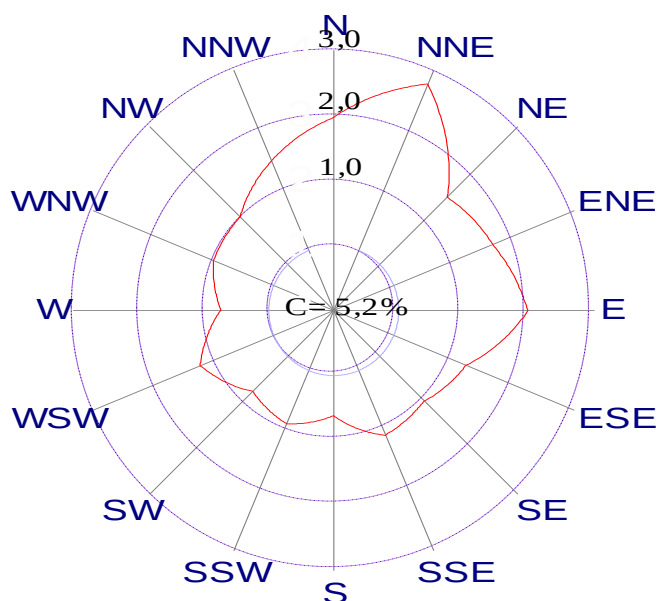
Slika 59 - Učestalost smjera vjetra [%] i srednje vrijednosti brzine vjetra [m/s] po smjerovima na mjernoj postaji 5-GOK natkriven određeni tijekom ljetnog razdoblja 2015. godine
