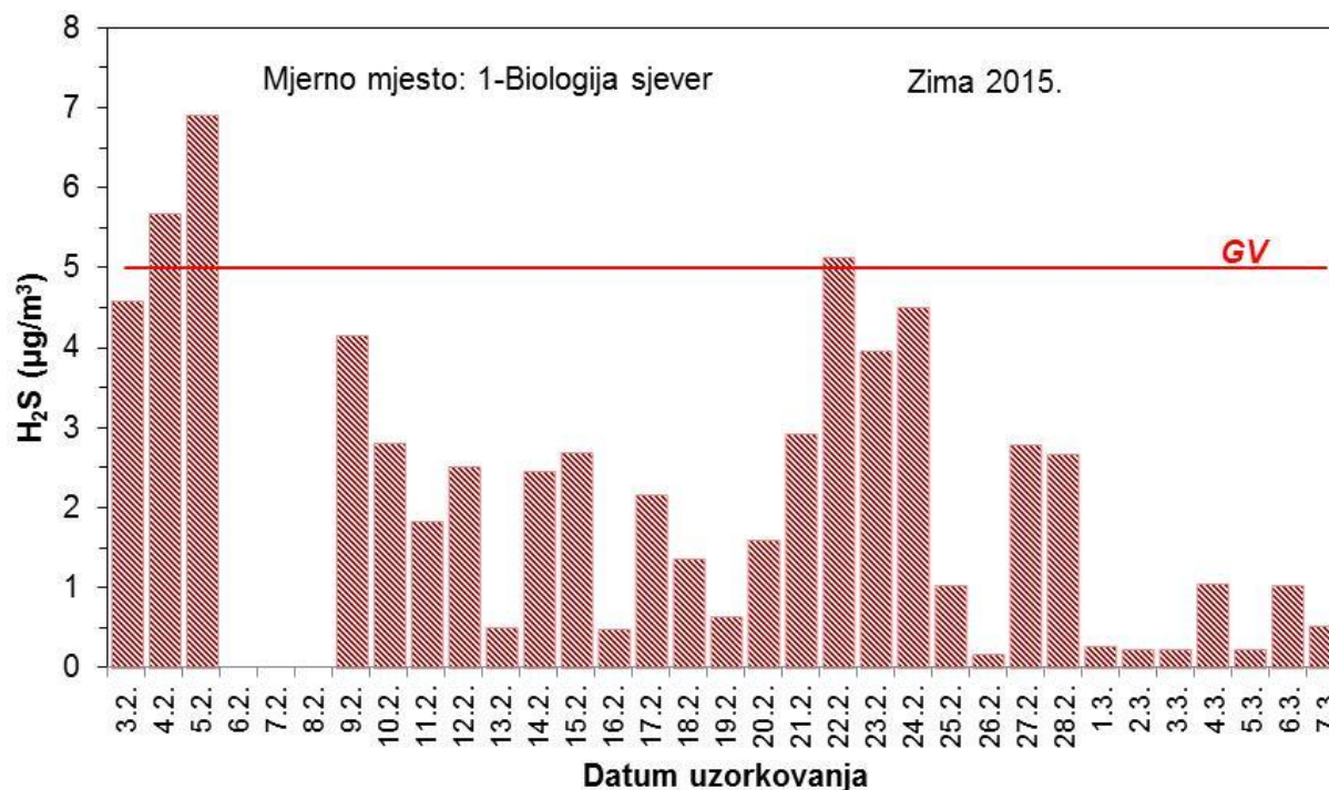
Slika 16 – Kretanje srednjih dnevnih koncentracija sumporovodika na mjernoj postaji 1 – Biologija sjever tijekom zimskog razdoblja mjerenja
