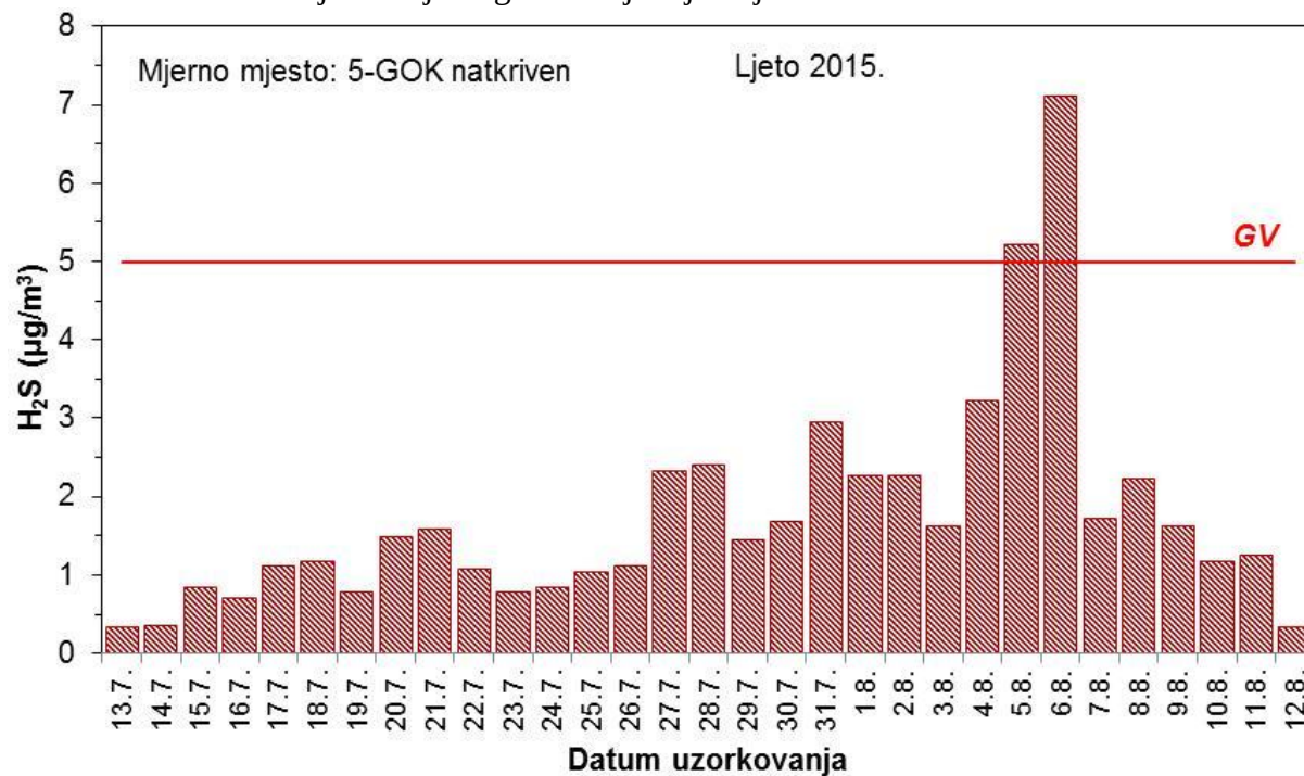
Slika 27 – Kretanje srednjih dnevnih koncentracija sumporovodika na mjernoj postaji 5 – GOK natkriven tijekom ljetnog razdoblja mjerenja
