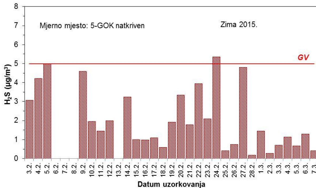
Slika 20 – Kretanje srednjih dnevnih koncentracija sumporovodika na mjernoj postaji 5 – GOK natkriven tijekom zimskog razdoblja mjerenja
