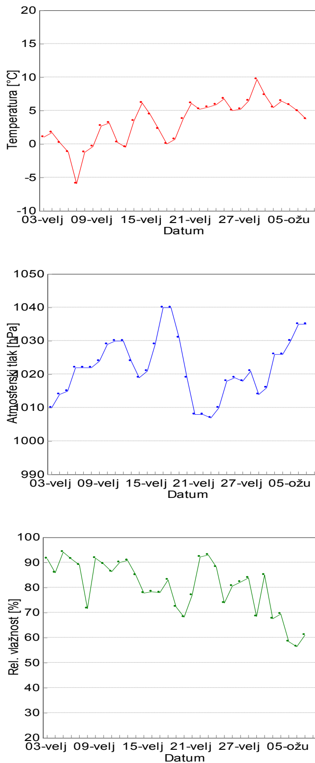
Slika 52 - Dnevni srednjaci temperature, tlaka i relativne vlažnosti na mjernoj postaji 4 - Mićevec određeni tijekom zimskog razdoblja 2015. godine
