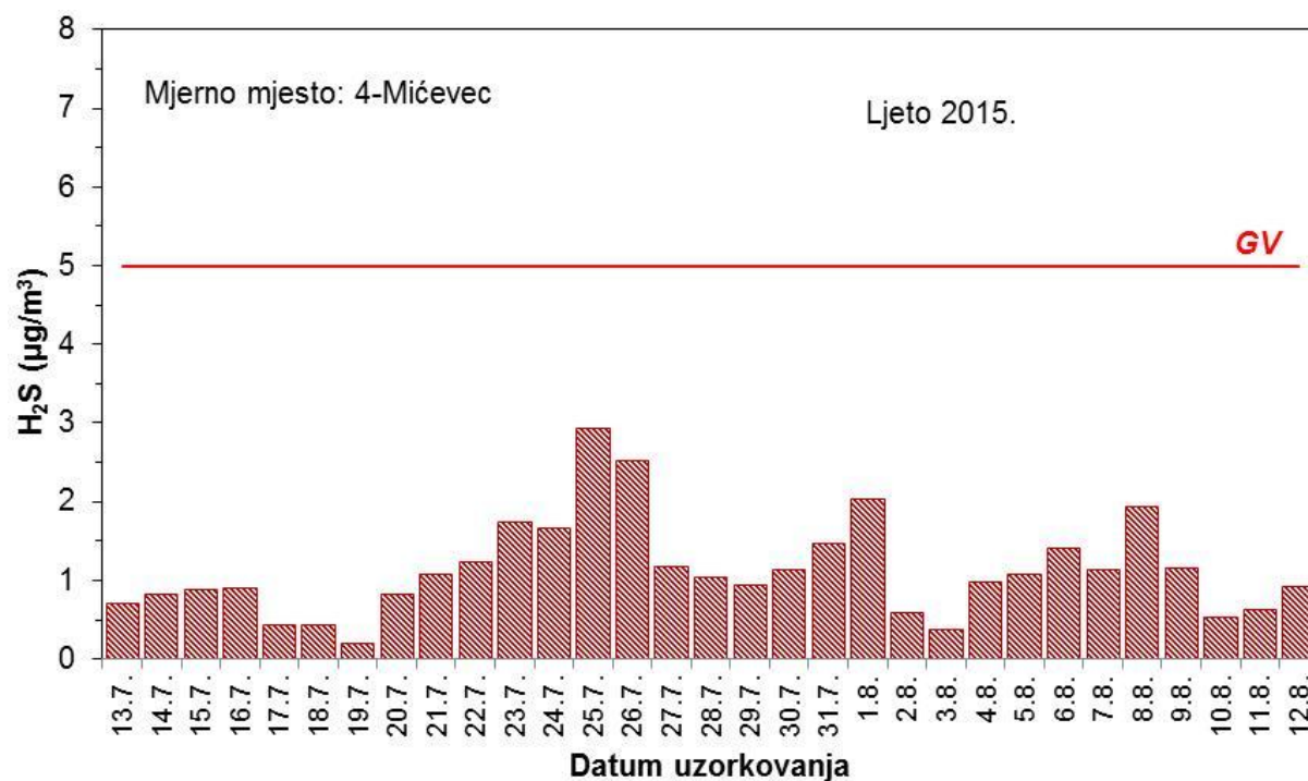
Slika 26 – Kretanje srednjih dnevnih koncentracija sumporovodika na mjernoj postaji 4 – Mičevac tijekom ljetnog razdoblja mjerenja
