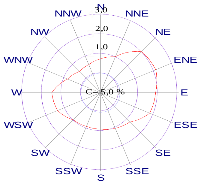
Slika 45 - Učestalost smjera vjetra [%] i srednje vrijednosti brzine vjetra [m/s] po smjerovima na mjernoj postaji 1 –Biologija sjever određeni tijekom zimskog razdoblja 2015. godine
