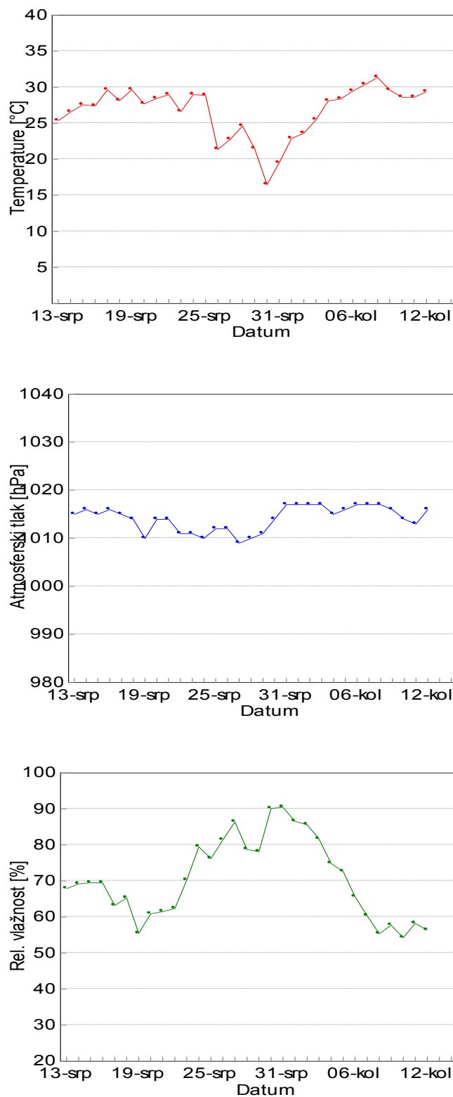
Slika 48 - Dnevni srednjaci temperature, tlaka i relativne vlažnosti na mjernoj postaji 1 –Biologija sjever određeni tijekom ljetnog razdoblja 2015. godine
