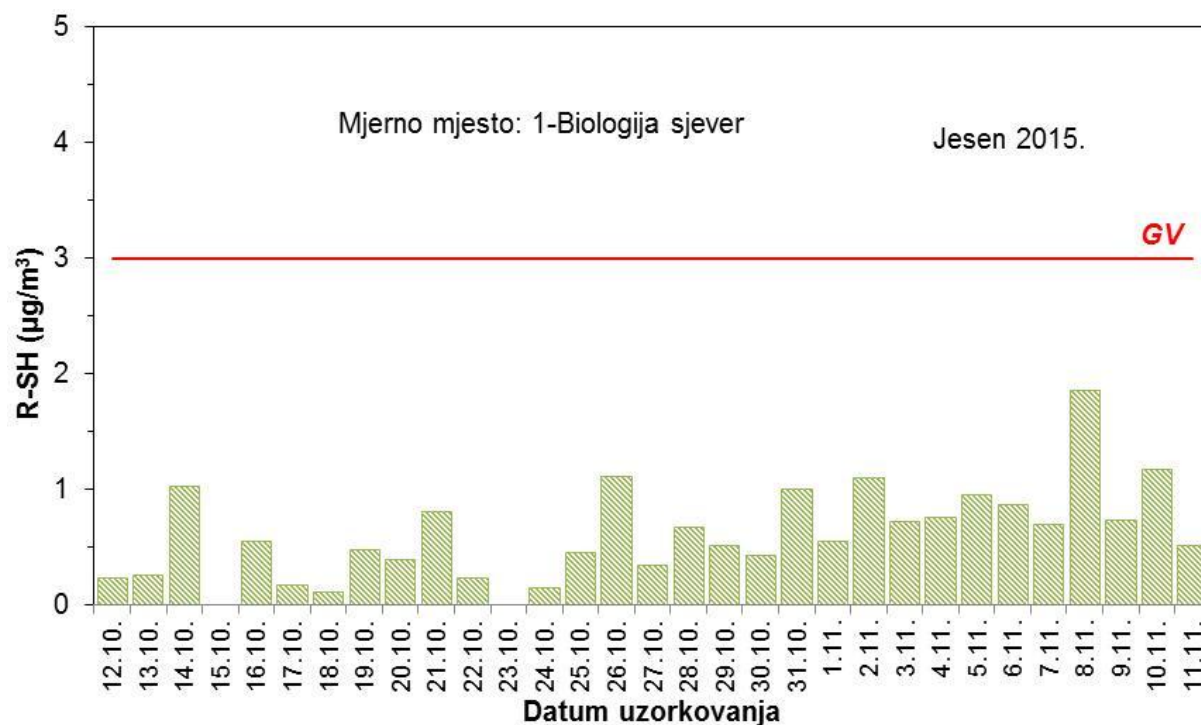
Slika 42 – Kretanje srednjih dnevnih koncentracija merkaptana na mjernoj postaji 1 – Biologija sjever tijekom jesenskog razdoblja mjerenja
