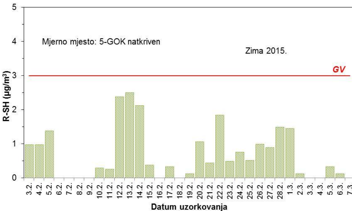
Slika 34 – Kretanje srednjih dnevnih koncentracija merkaptana na mjernoj postaji 5 – GOK natkriven tijekom zimskog razdoblja mjerenja
