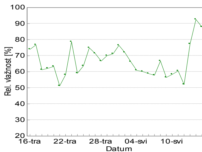
Slika 46 - Dnevni srednjaci temperature, tlaka i relativne vlažnosti na mjernoj postaji 1 –Biologija sjever određeni tijekom proljetnog razdoblja 2015. godine
