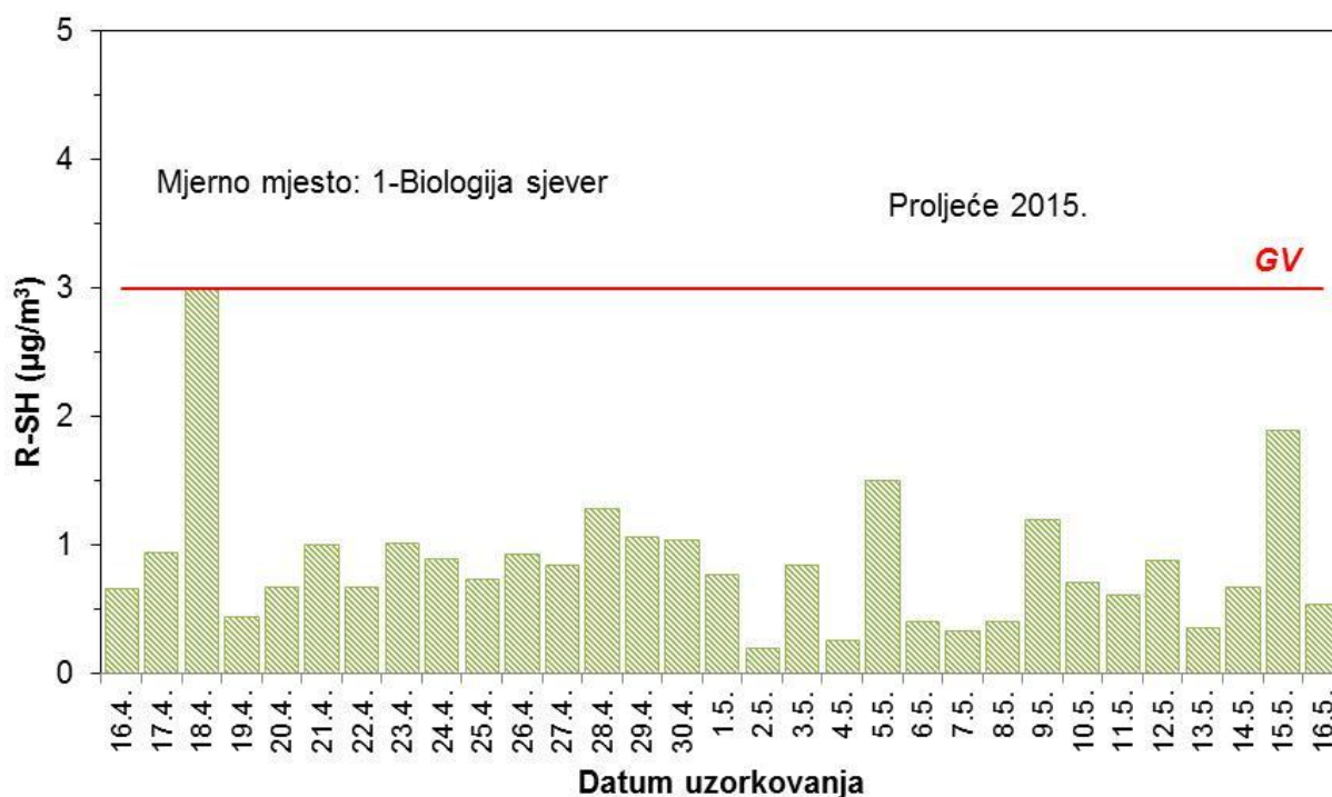
Slika 35 – Kretanje srednjih dnevnih koncentracija merkaptana na mjernoj postaji 1 – Biologija sjever tijekom proljetnog razdoblja mjerenja
