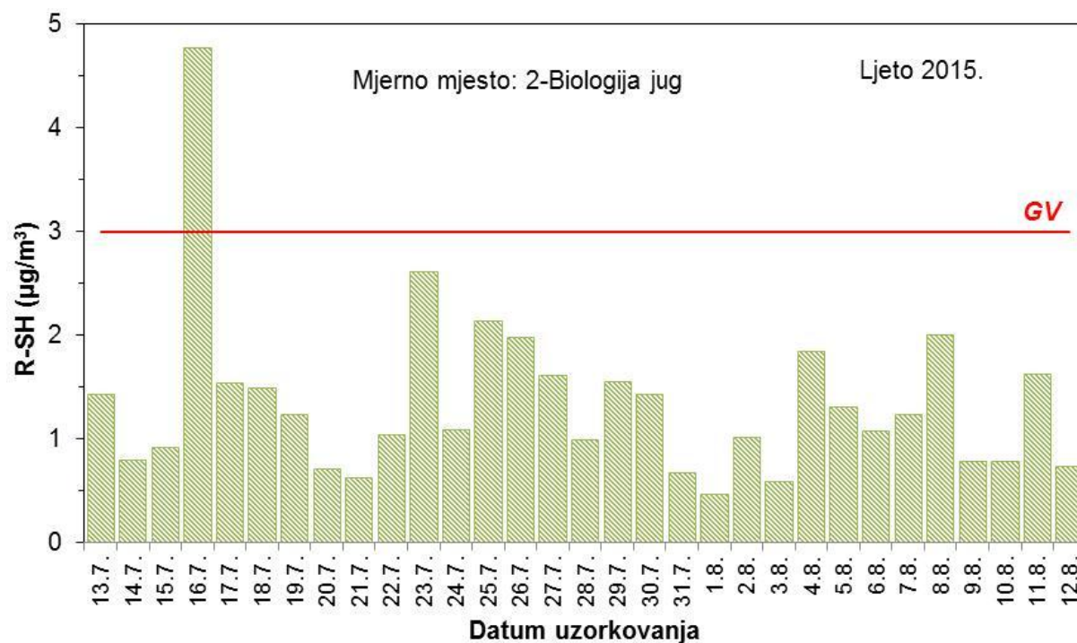
Slika 38 – Kretanje srednjih dnevnih koncentracija merkaptana na mjernoj postaji 2 – Biologija jug tijekom ljetnog razdoblja mjerenja
