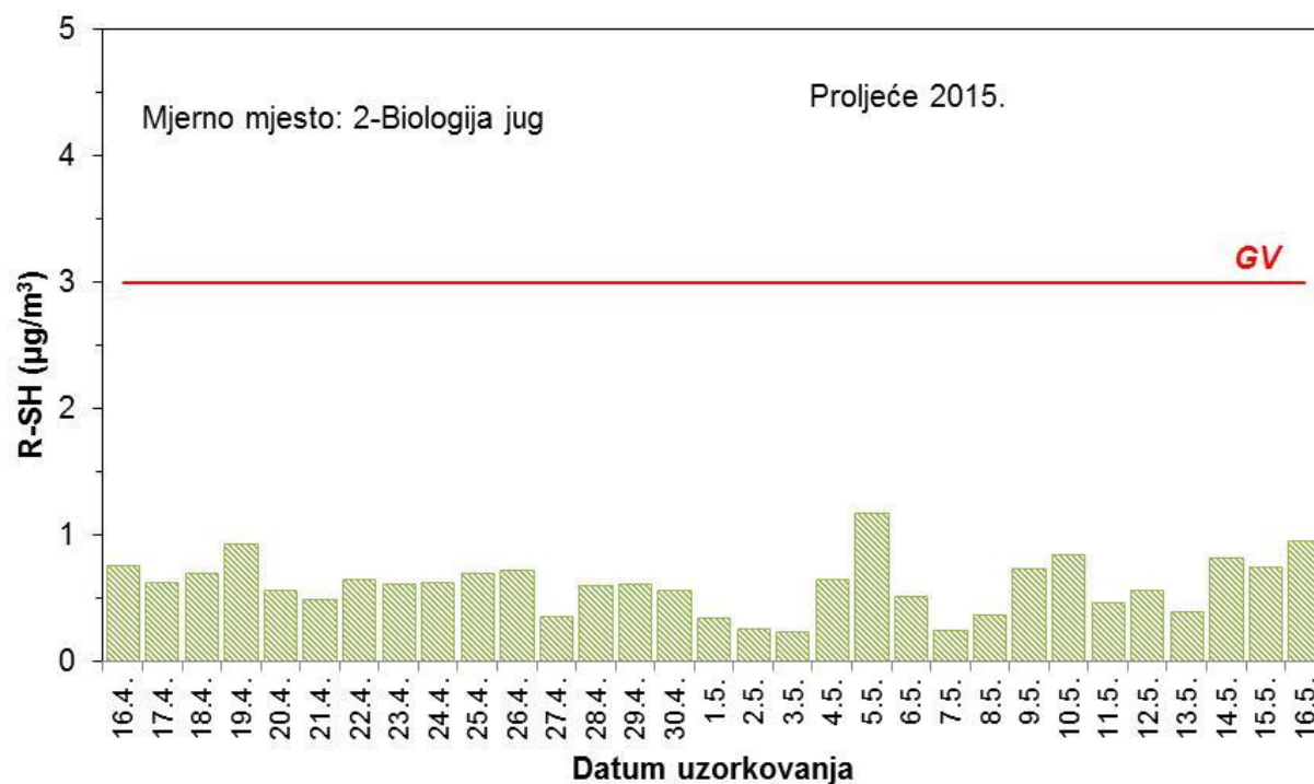
Slika 36 – Kretanje srednjih dnevnih koncentracija merkaptana na mjernoj postaji 2 – Biologija jug tijekom proljetnog razdoblja mjerenja
