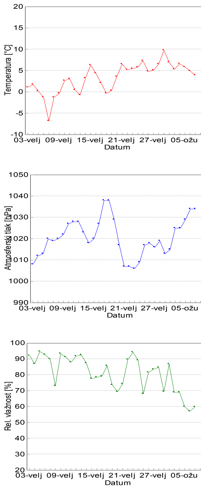
Slika 44 - Dnevni srednjaci temperature, tlaka i relativne vlažnosti na mjernoj postaji 1 –Biologija sjever određeni tijekom zimskog razdoblja 2015. godine
