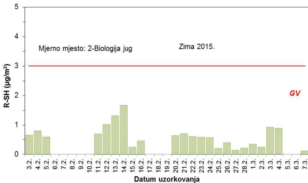
Slika 31 – Kretanje srednjih dnevnih koncentracija merkaptana na mjernoj postaji 2 – Biologija jug tijekom zimskog razdoblja mjerenja
