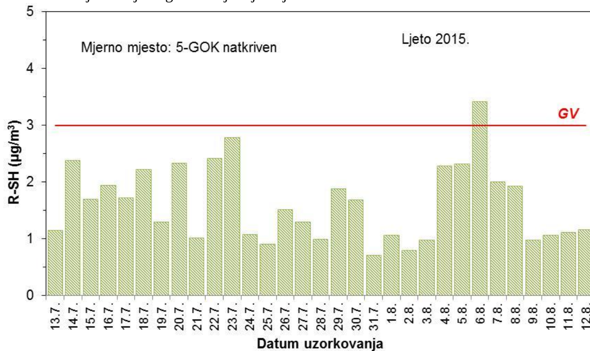
Slika 41 – Kretanje srednjih dnevnih koncentracija merkaptana na mjernoj postaji 5 – GOK natkriven tijekom ljetnog razdoblja mjerenja
