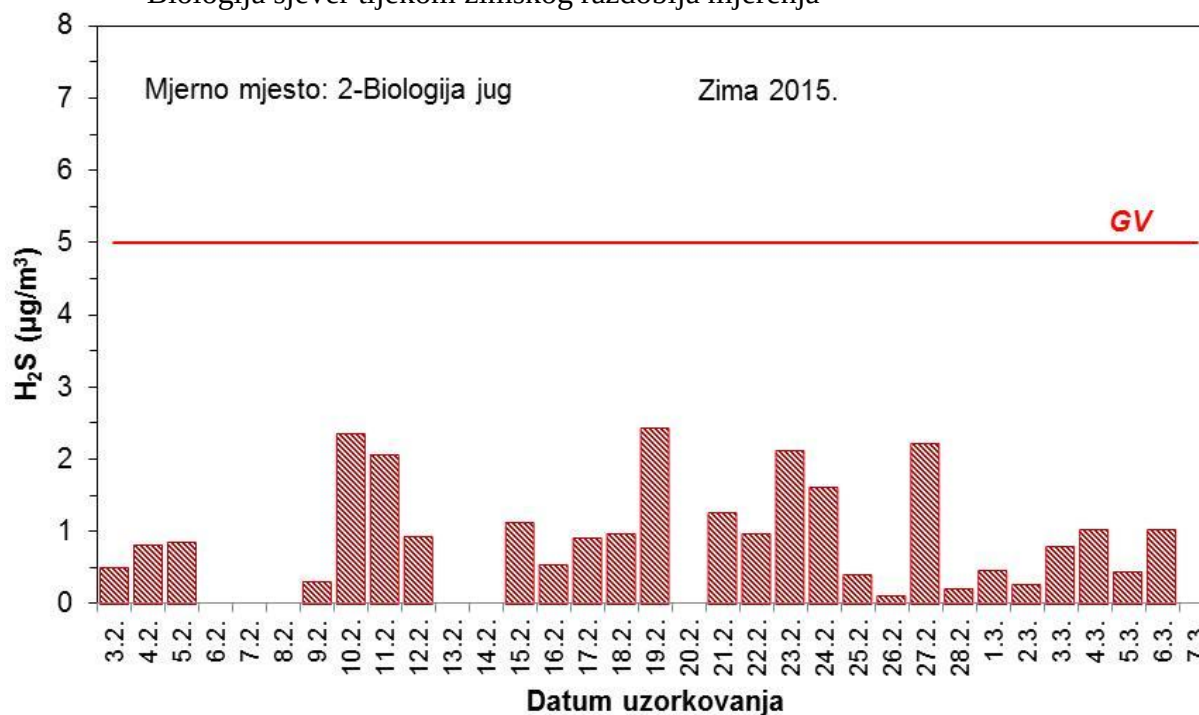
Slika 17 – Kretanje srednjih dnevnih koncentracija sumporovodika na mjernoj postaji 2 – Biologija jug tijekom zimskog razdoblja mjerenja
