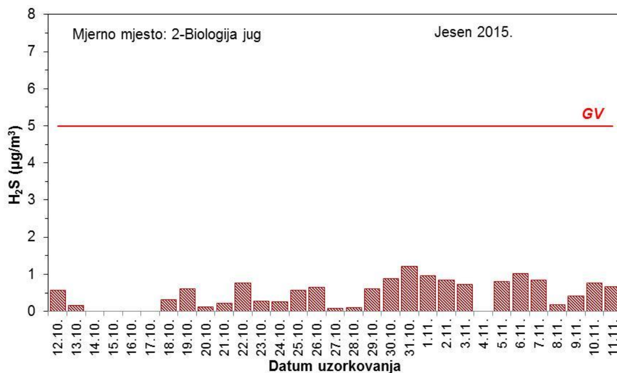
Slika 29 – Kretanje srednjih dnevnih koncentracija sumporovodika na mjernoj postaji 2 – Biologija jug tijekom jesenskog razdoblja mjerenja
