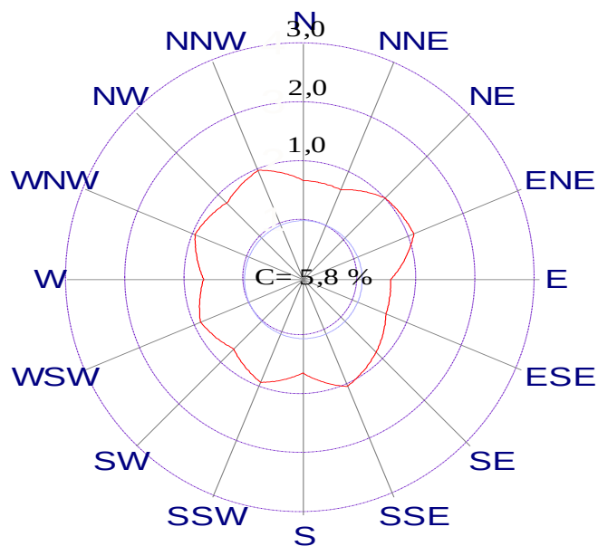
Slika 55 - Učestalost smjera vjetra [%] i srednje vrijednosti brzine vjetra [m/s] po smjerovima na mjernejoj postaji 4 – Mićevec određeni tijekom ljetnog razdoblja 2015. godine
