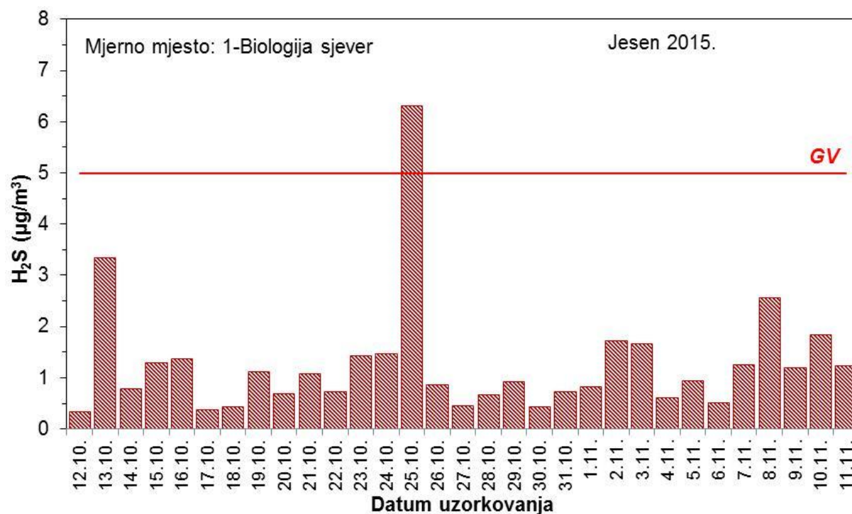
Slika 28 – Kretanje srednjih dnevnih koncentracija sumporovodika na mjernoj postaji 1 – Biologija sjever tijekom jesenskog razdoblja mjerenja
