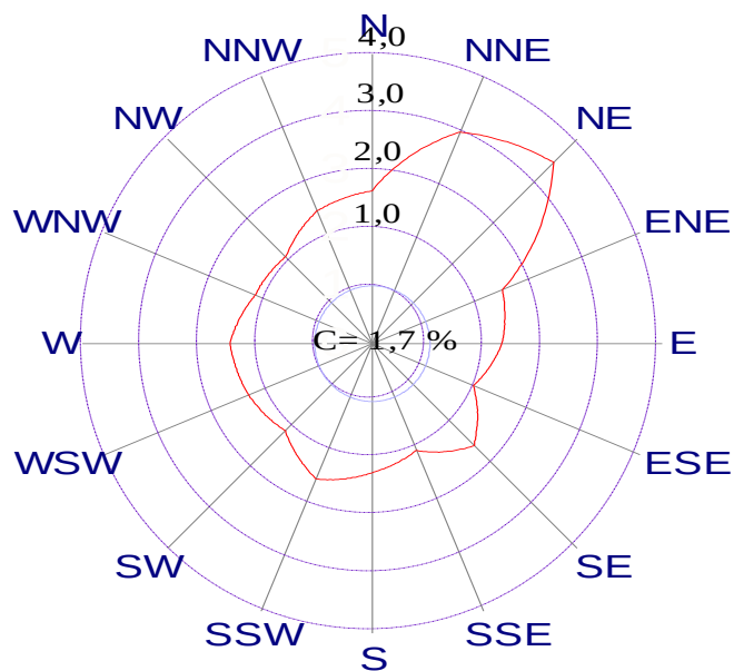
Slika 51 - Učestalost smjera vjetra [%] i srednje vrijednosti brzine vjetra [m/s] po smjerovima na mjernoj postaji 1 –Biologija sjever određeni tijekom jesenskog razdoblja 2015. godine
