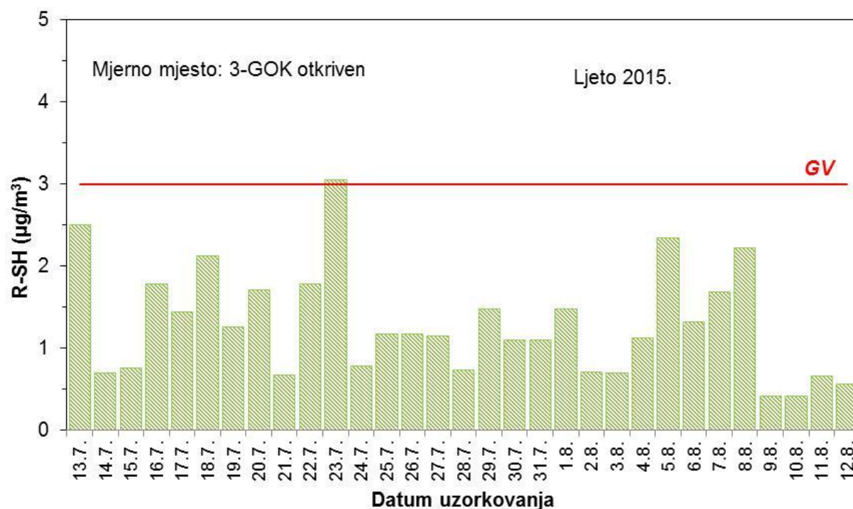
Slika 39 – Kretanje srednjih dnevnih koncentracija merkaptana na mjernoj postaji 3 – GOK otkriven tijekom ljetnog razdoblja mjerenja
