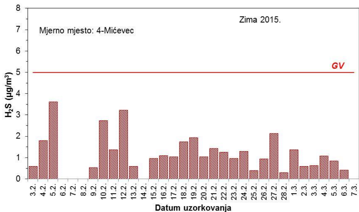
Slika 19 – Kretanje srednjih dnevnih koncentracija sumporovodika na mjernoj postaji 4 – Mićevec tijekom zimskog razdoblja mjerenja
