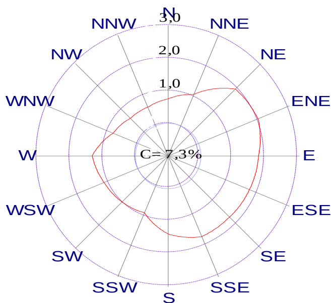
Slika 57 - Učestalost smjera vjetra [%] i srednje vrijednosti brzine vjetra [m/s] po smjerovima na mjernoj postaji 5-GOK natkriven određeni tijekom zimskog razdoblja 2015. godine
