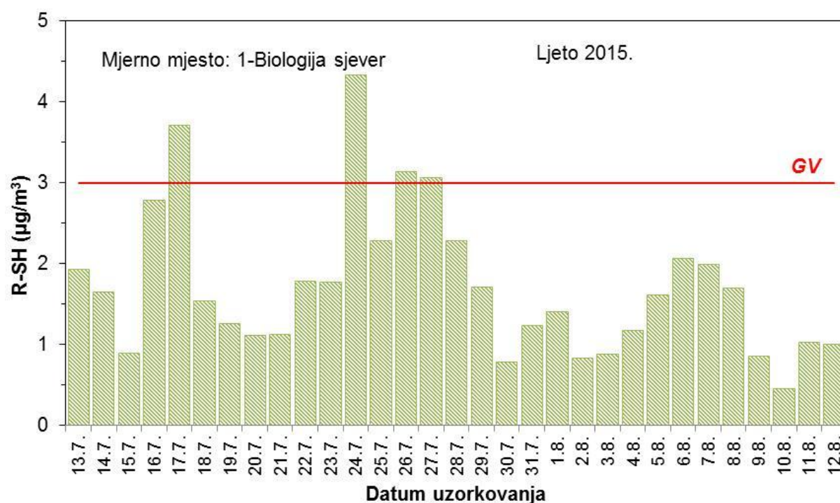
Slika 37 – Kretanje srednjih dnevnih koncentracija merkaptana na mjernoj postaji 1 – Biologija sjever tijekom ljetnog razdoblja mjerenja
