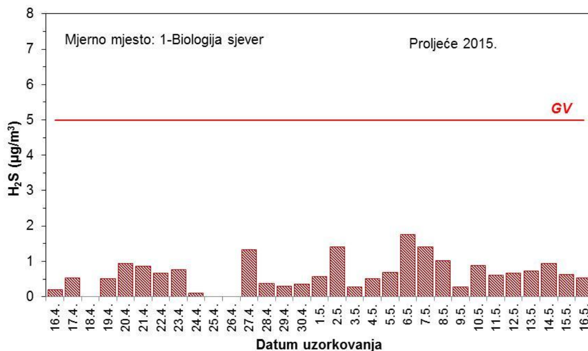
Slika 21 – Kretanje srednjih dnevnih koncentracija sumporovodika na mjernoj postaji 1 – Biologija sjever tijekom proljetnog razdoblja mjerenja
