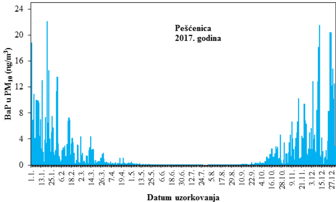
Slika 1 – Kretanje srednjih dnevnih koncentracija BaP u frakciji lebdećih čestica PM 10 tijekom 2017. godine na mjernoj postaji na Peščenici
