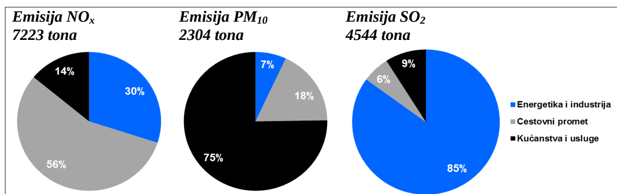
Sl. 6-2: Godišnje emisije i udjeli pojedinih sektora u emisijama \text{NO}_x , \text{PM}_{10} i \text{SO}_2
