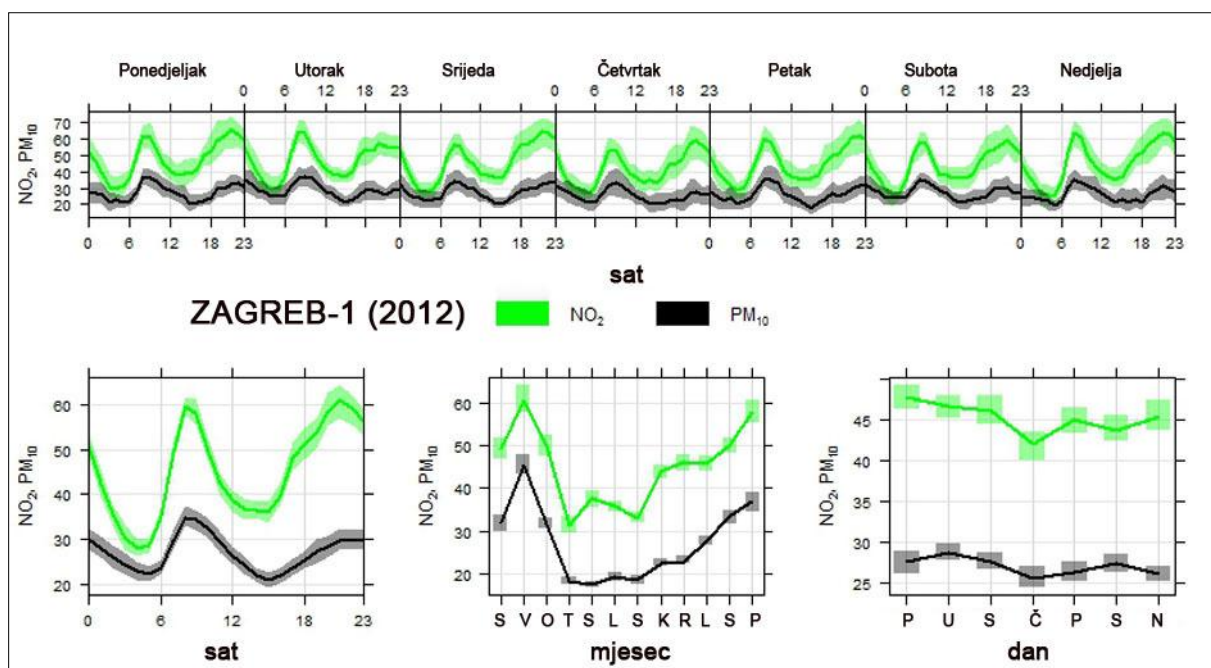
Sl. 6-10: Vremenska promjenjivost koncentracija \text{NO}_2 i \text{PM}_{10} na lokacijama Ksaverska cesta i Zagreb-1 u 2012.
