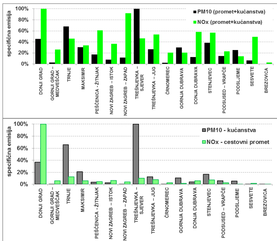
Sl. 6-6: Relativne vrijednosti specifičnih emisija \text{NO}_x i \text{PM}_{10} (ukupno i za dominantne izvore)
