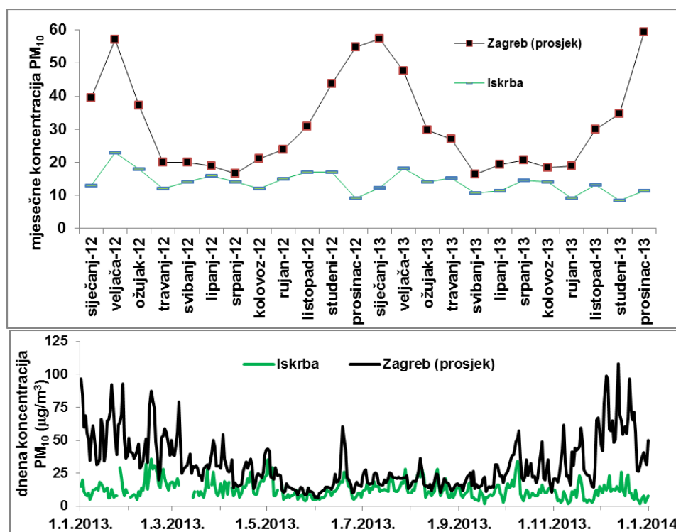
Sl. 6-13: Mjesečne i dnevne koncentracije \text{PM}_{10} na ruralnom području (Iskra, Slovenija) i na području grada Zagreba
